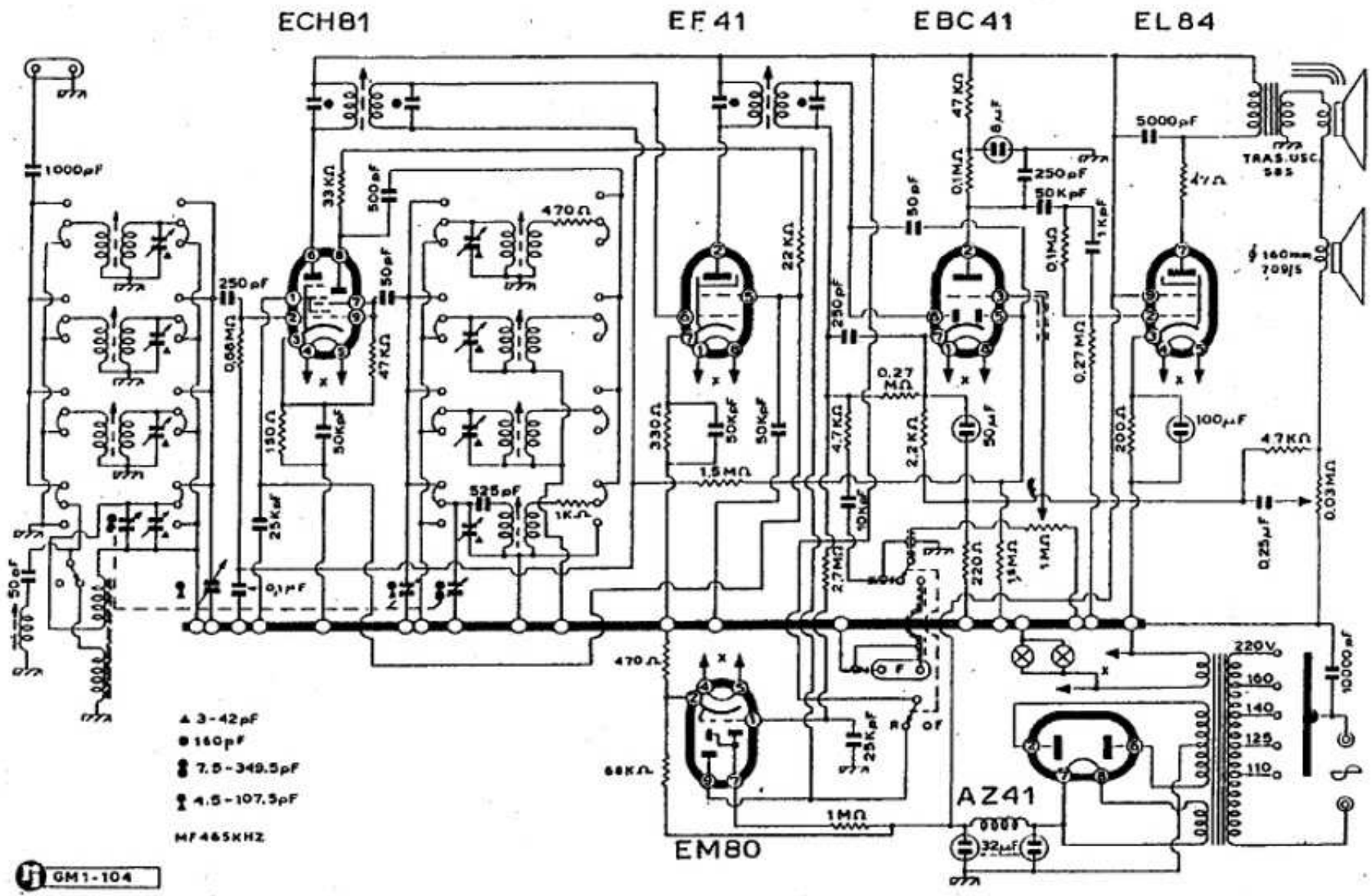
Allocchio Bacchini - Mod. 955/TA ediz. C
